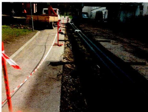
24.att. Cauruļvadu montāža uz pagaidu balstiem virs demontējām siltumtīklu caurulēm
