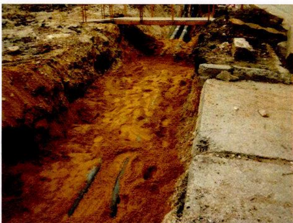
9.att. Cauruļvadu apbērsšana ar smilti II posms
