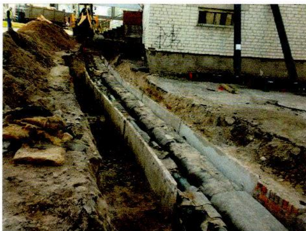
23.att. Tranšejas atrakšana un esošo cauruļu demontāža posmā no katlu mājas uz slimnīcas pusi
